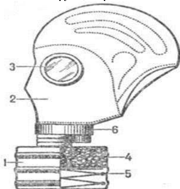
Рис. 1. Фильтрующий противогаз
